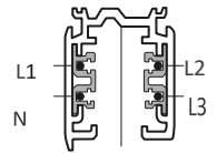
Трехфазный шинопровод
