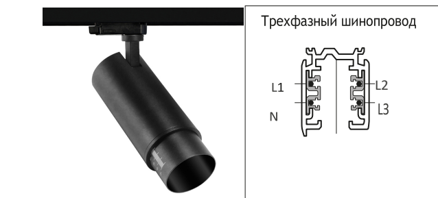
Правильная установка
