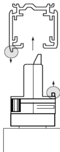
Правильная установка
