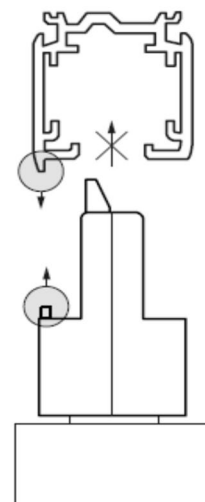
Неправильная установка
